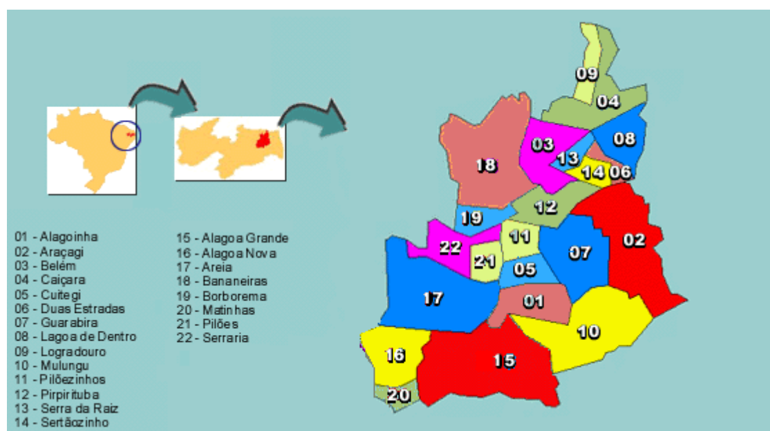
Fig. 1. Nordeste da Paraíba com suas 22 microrregiões.
